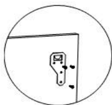
Схема крепления навесной пластины (рис.2)
