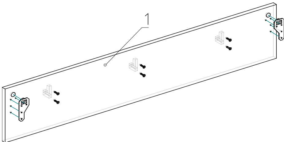
Схема сборки вешалки (рис.1)
