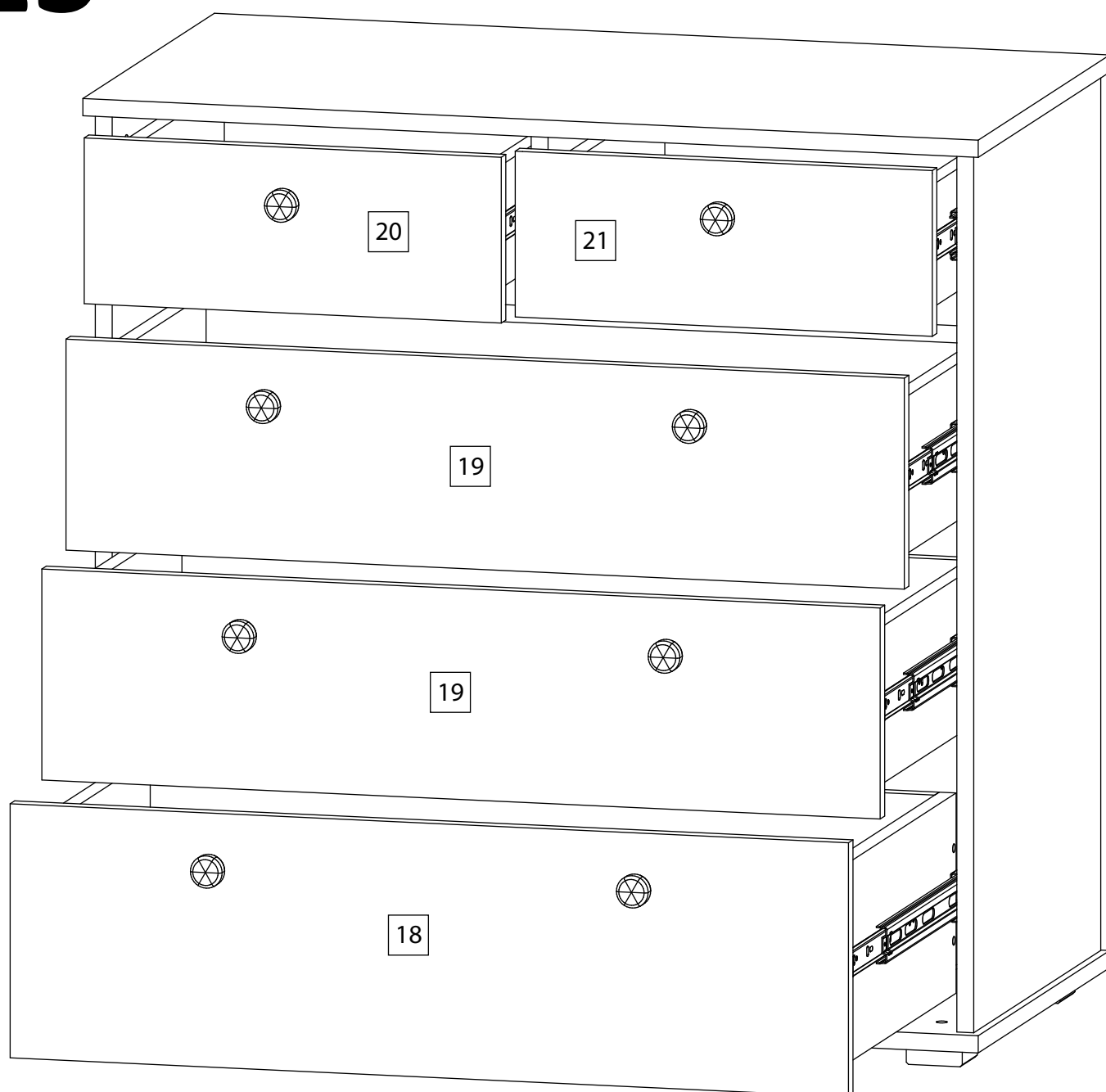
Установка ящика
