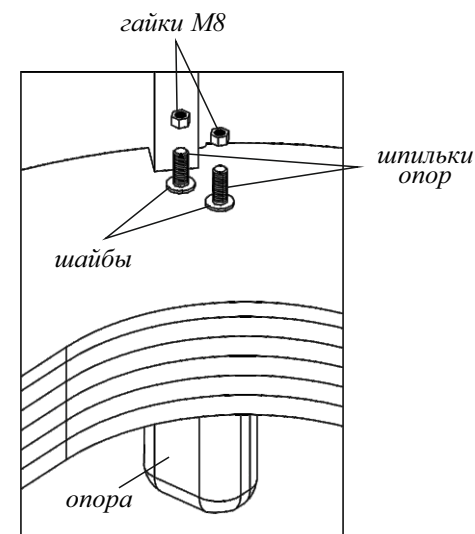
Схема установки опор (под сиденьем)
